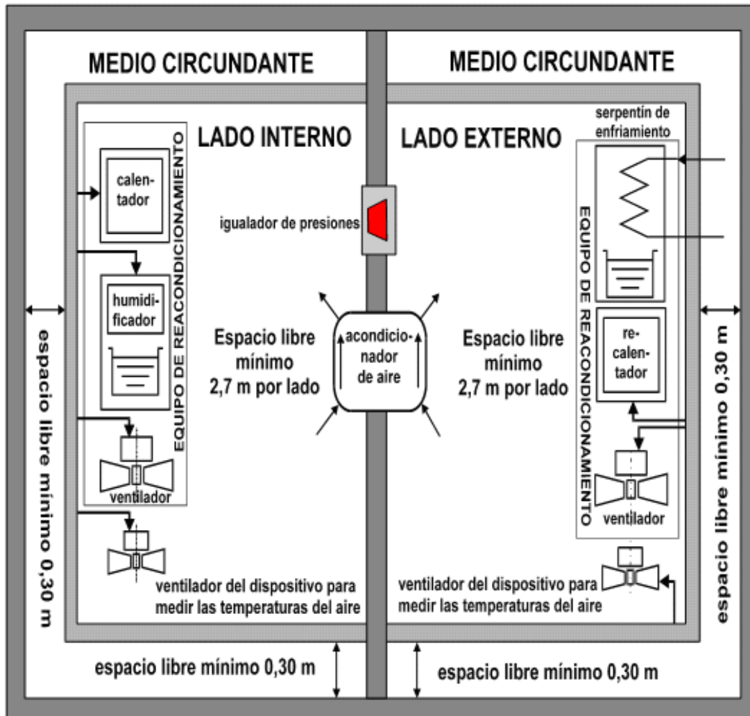
Figura 1. Calorímetro de cuarto tipo ambiente balanceado
